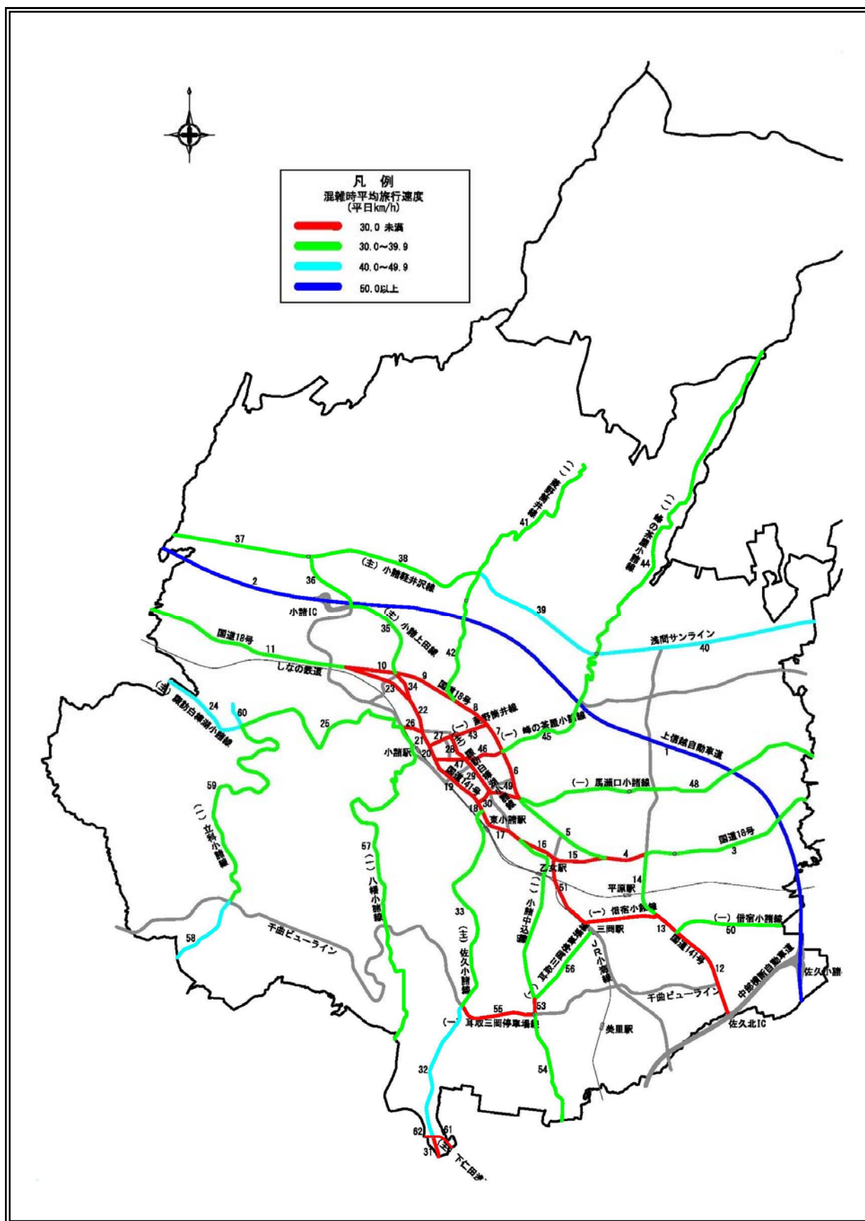
図 6-1 混雑時平均旅行速度分布図 (平成 27(2015) 年)
