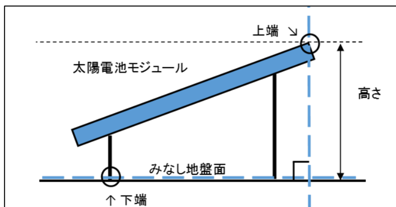
【図 1】太陽電池モジュールの高さ
