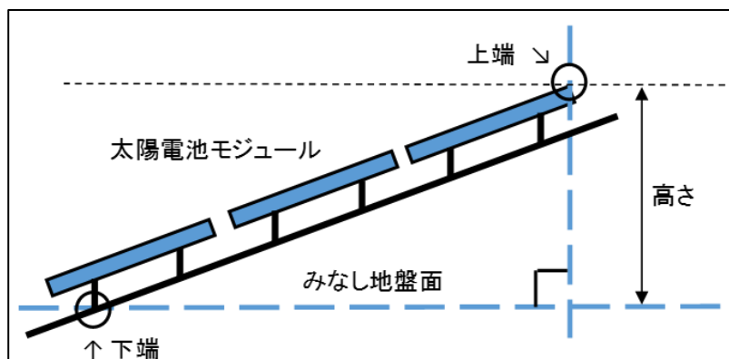
【図 2】一段の土地に連続して設置される太陽電池モジュールの高さ
